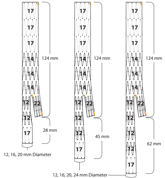
ZFEN-D-(12)(16)(20)(24)-(28)(45)(62)-124
