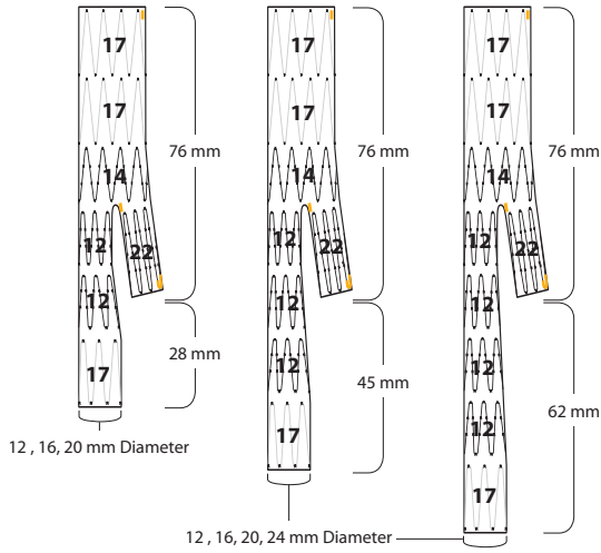
ZFEN-D-(12)(16)(20)(24)-(28)(45)(62)-76
