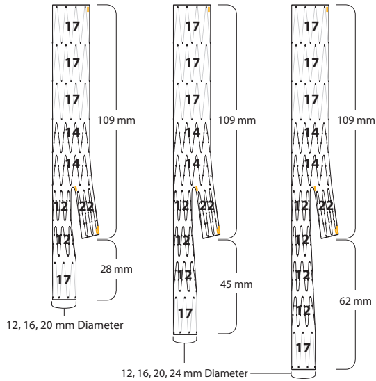
ZFEN-D-(12)(16)(20)(24)-(28)(45)(62)-109
